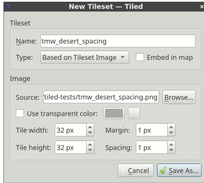
Abb. 3: Neues Tileset
