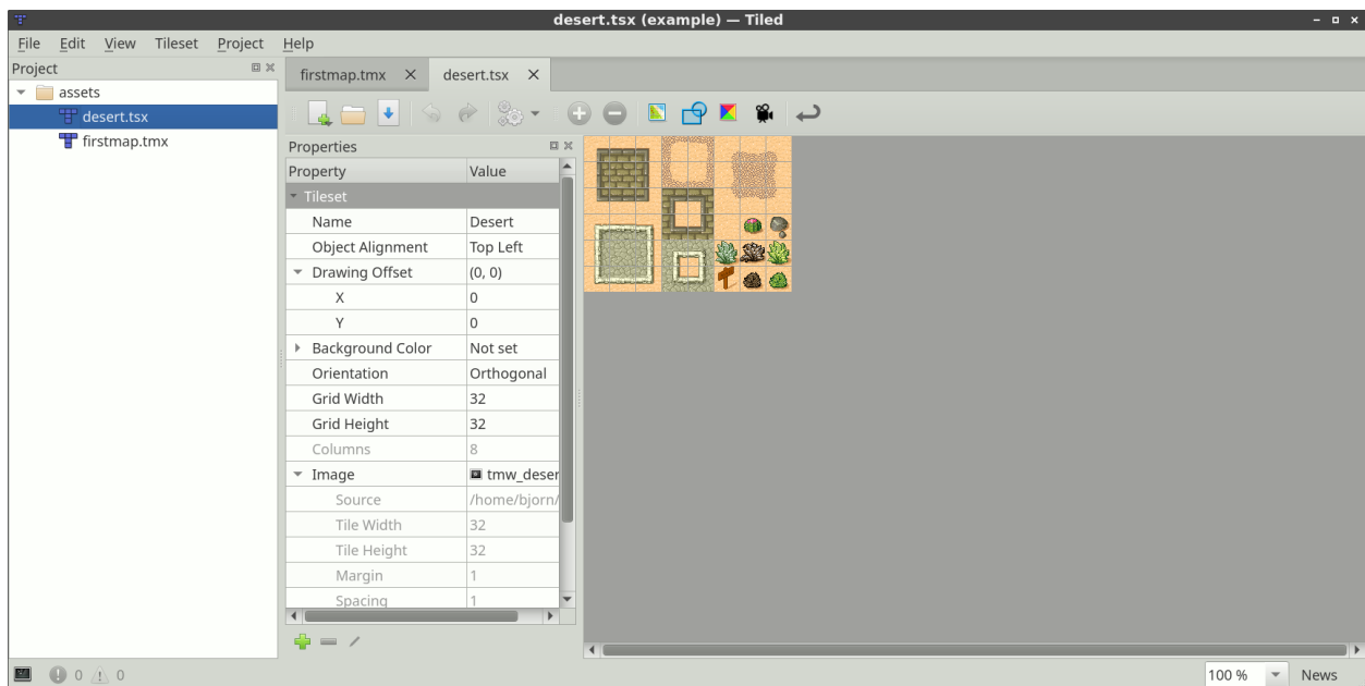
Abb. 4: Erzeugtes Tileset
